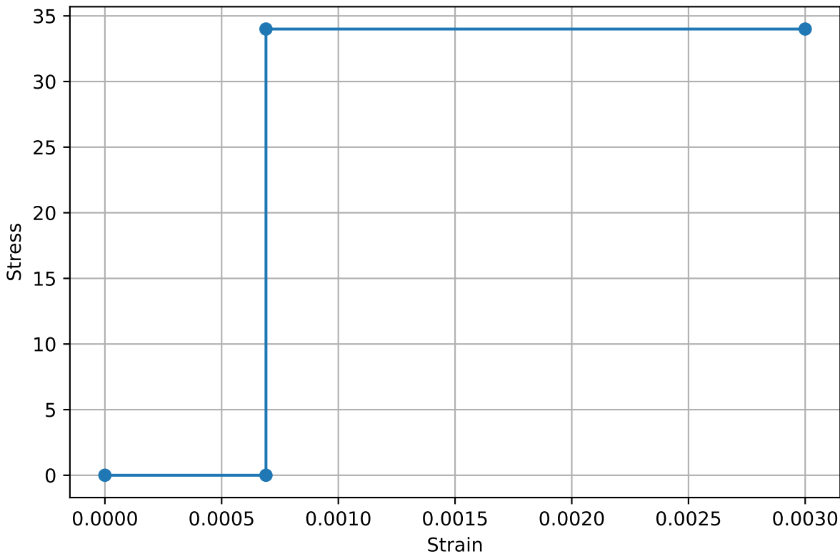
40 MPa Conc [2300 kg/m 3 ] (NZS3101:2006) - Ultimate Profile
